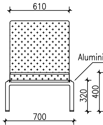
A Front view 正视图 SCALE 1:15
