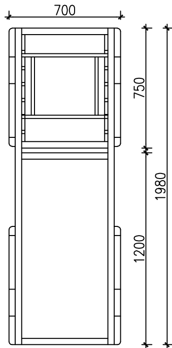
C Top view 俯视图 SCALE 1:15
