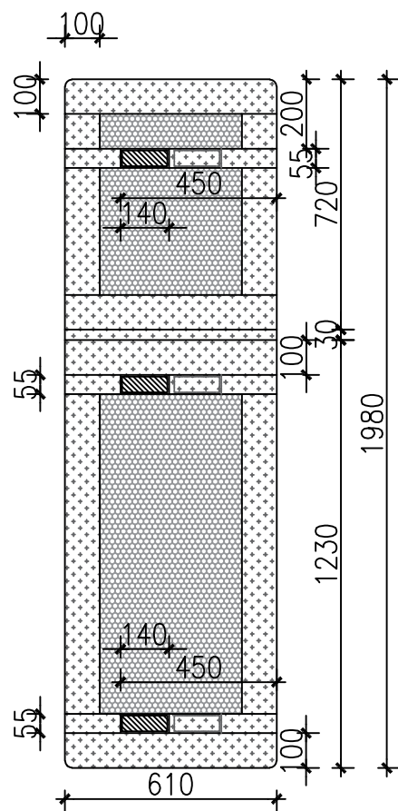
C Top view 俯视图 SCALE 1:15
